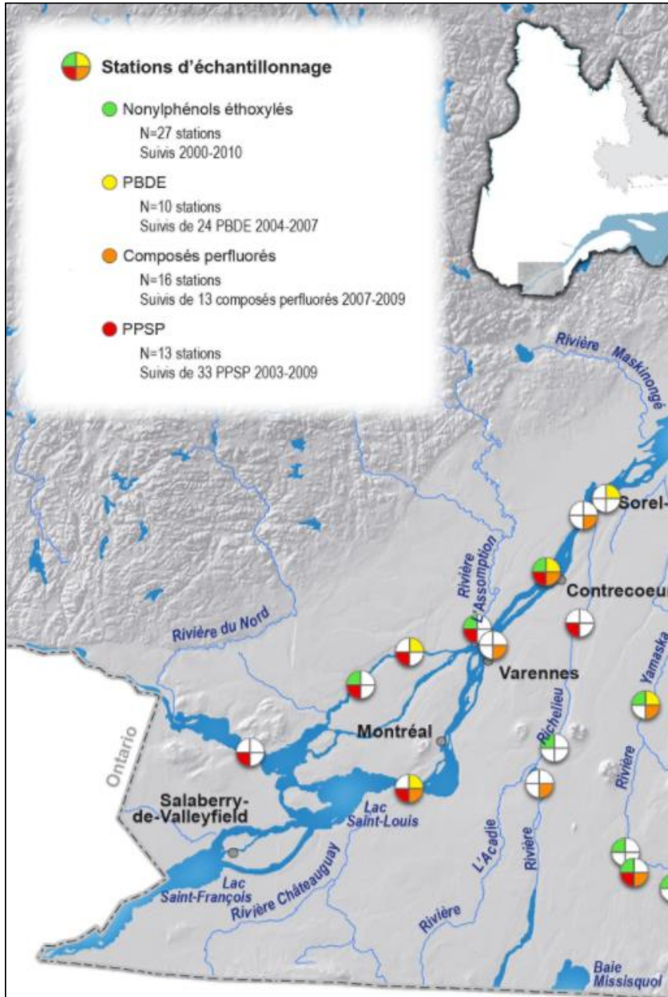
Figure 12 — Présence de contaminants émergents dans les cours d'eau de la zone Haut-Saint-Laurent - Grand Montréal (Source : MDDELCC, 2013)
