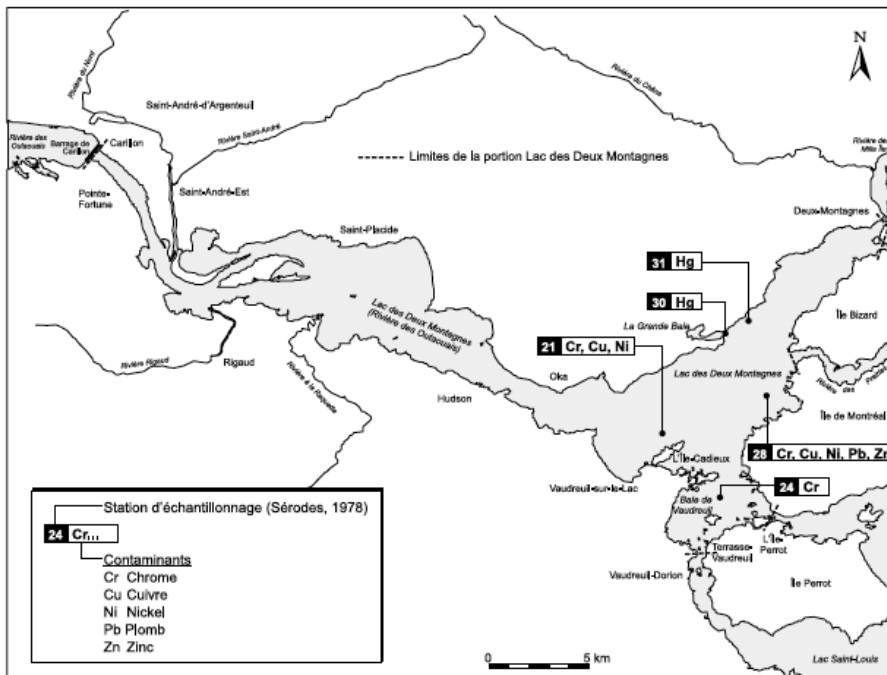
Figure 6 : Dégradations localisées dans le secteur Lac des Deux Montagnes (Robitaille, 1999)
