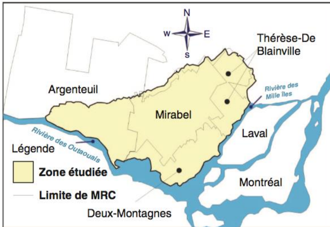
Figure 15 — Secteur de Mirabel étudié par la Commission géologique du Canada (source : Savard et al., 2013)
